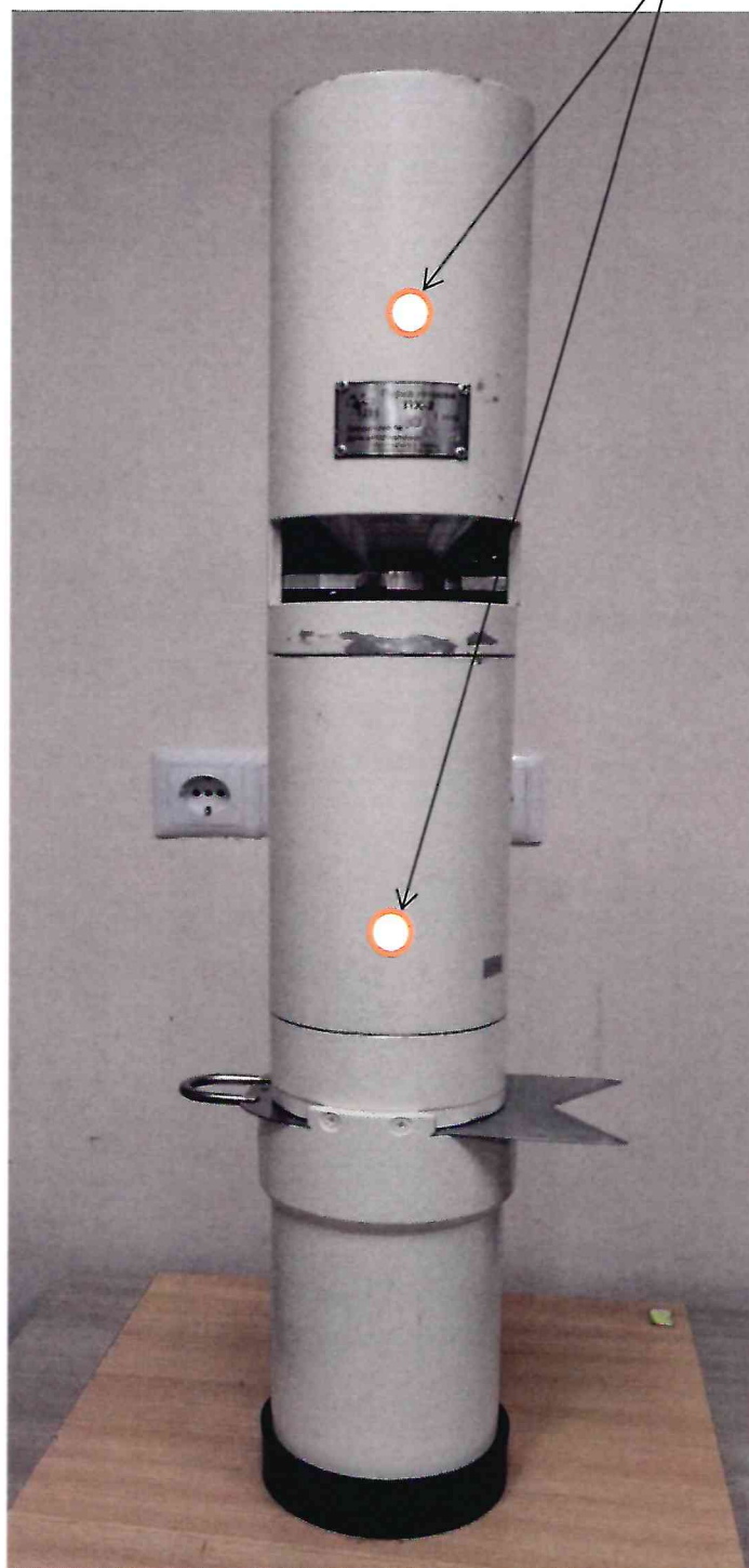
Рисунок 2.1 - Фотография с указанием места нанесения знака поверки (наклейки) на пурку литровую рабочую с падающим грузом ПХ-2 № 16129
