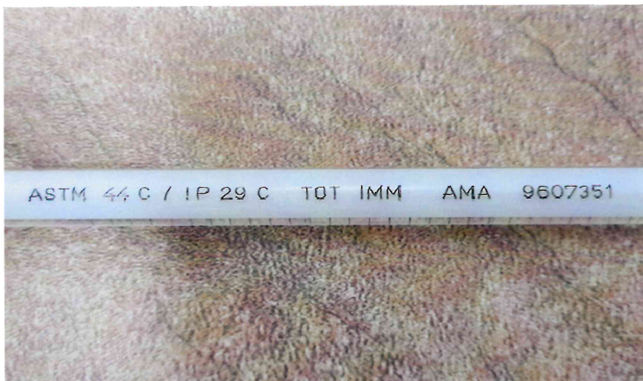
Рисунок 1.2 – Фотография маркировки термометра стеклянного ASTM 44C/IP29C № 9607351
