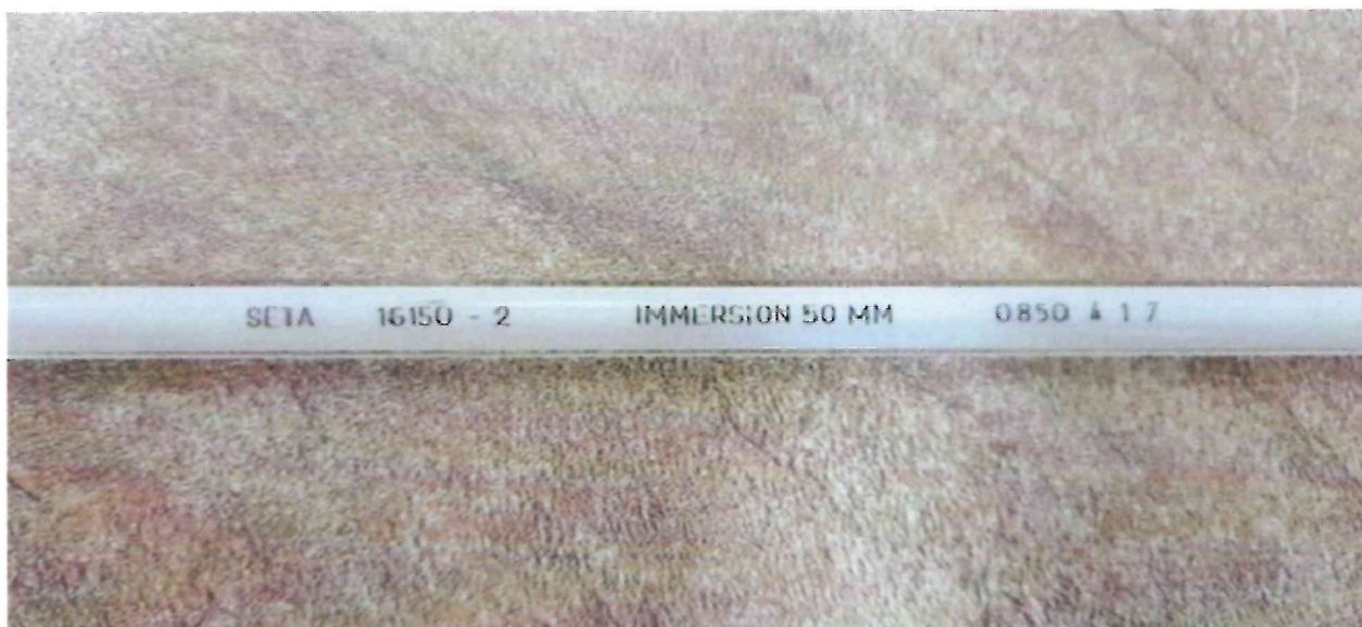
Рисунок 1.2 – Фотография маркировки термометра стеклянного SETA 16150-2 № 0850417
