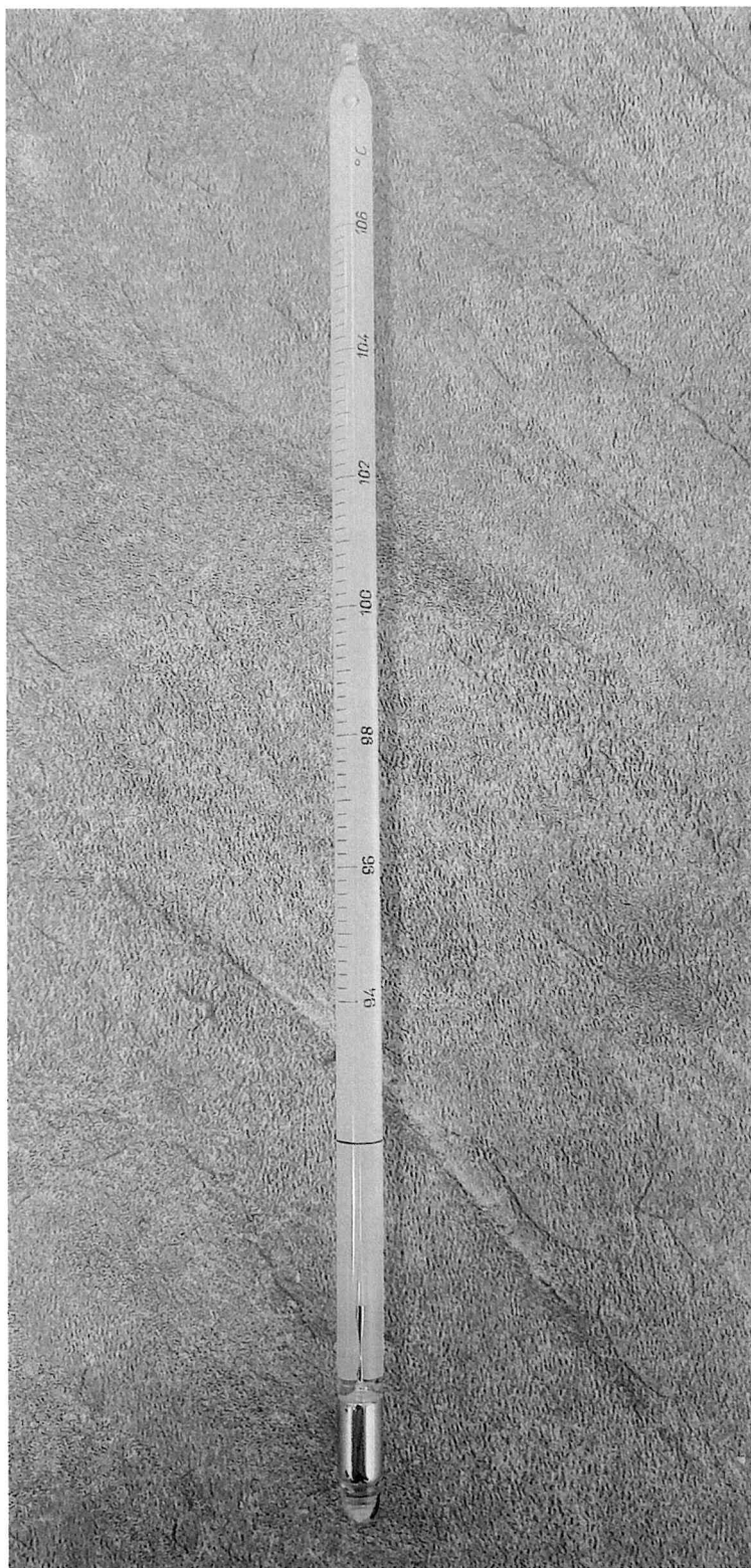
Рисунок 1.1 – Фотография общего вида термометра стеклянного SETA 16150-2 № 0850416
