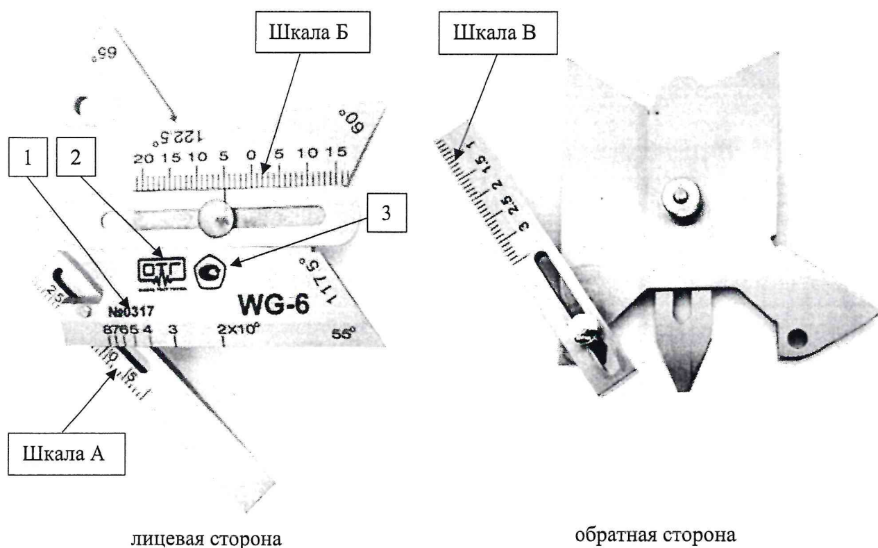
Рисунок 8 – Общий вид шаблона сварщика универсального WG, исполнение WG-6 (лицевая и обратная сторона)
