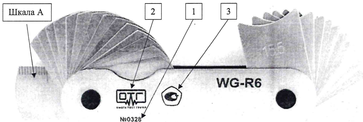
Рисунок 18 – Общий вид шаблона сварщика универсального WG, исполнение WG-R5 1 – место нанесения заводского номера; 2 – логотип изготовителя; 3 – место нанесения знака утверждения типа
