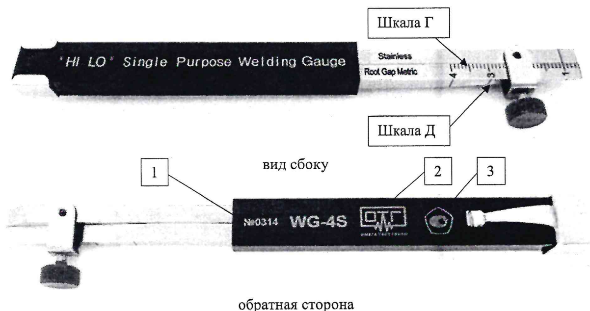
Рисунок 5 – Общий вид шаблона сварщика универсального WG, исполнение WG-4S 1 – место нанесения заводского номера; 2 – логотип изготовителя; 3 – место нанесения знака утверждения типа
