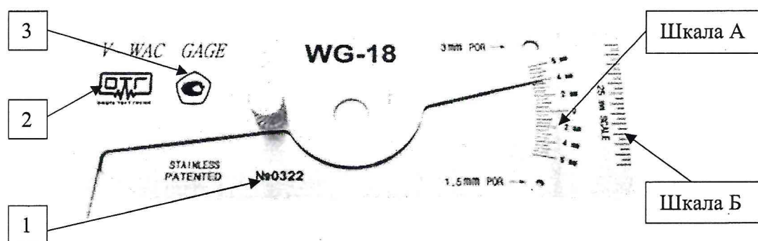
Рисунок 13 – Общий вид шаблона сварщика универсального WG, исполнение WG-18
