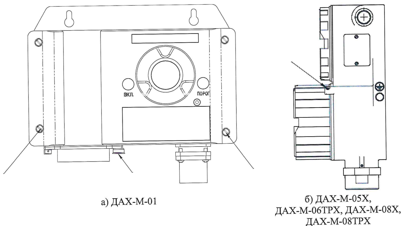
Рисунок 2 - Схема пломбировки газоанализаторов от несанкционированного доступа, обозначение мест для нанесения оттисков клейм (показаны стрелками)
