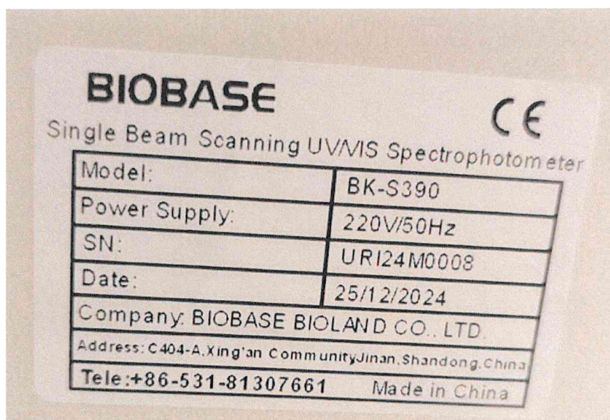
Рисунок 1.2 – Фотография маркировки спектрофотометра BK-S390 № URI24M0008
