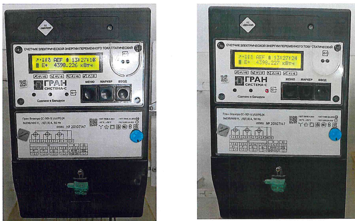
Рисунок 1.2 – Фотографии счётчиков, входящих в состав измерительных каналов АСКУЭ (изображения носят иллюстративный характер)
