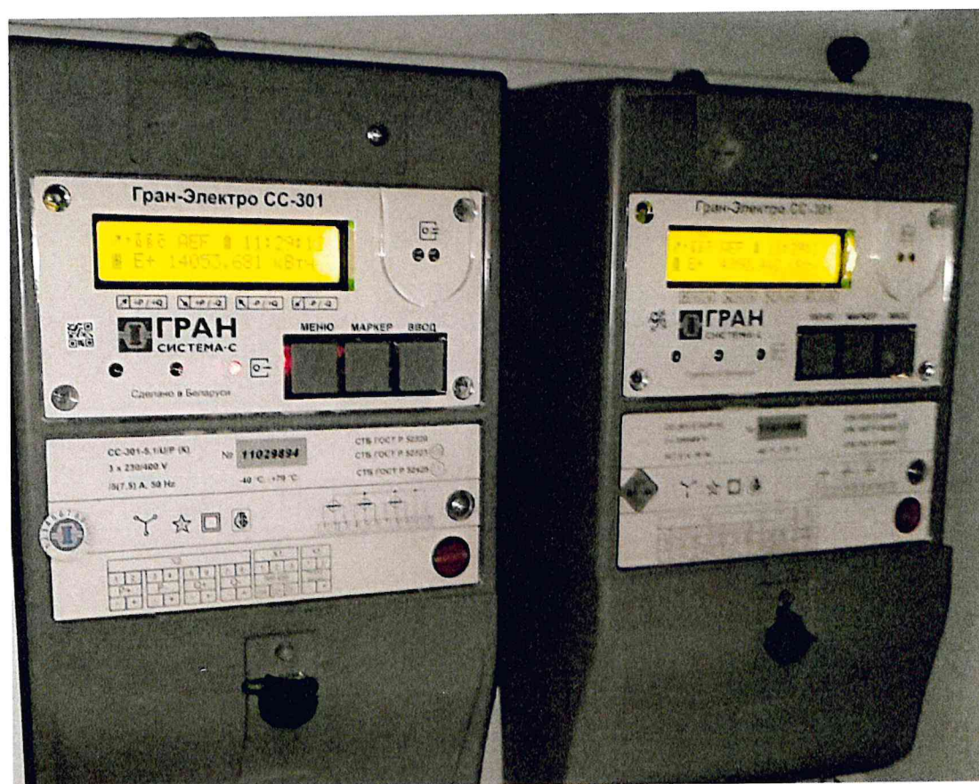
Рисунок 1.2 – Фотография общего вида счетчиков электрической энергии (изображение носит иллюстративный характер)
