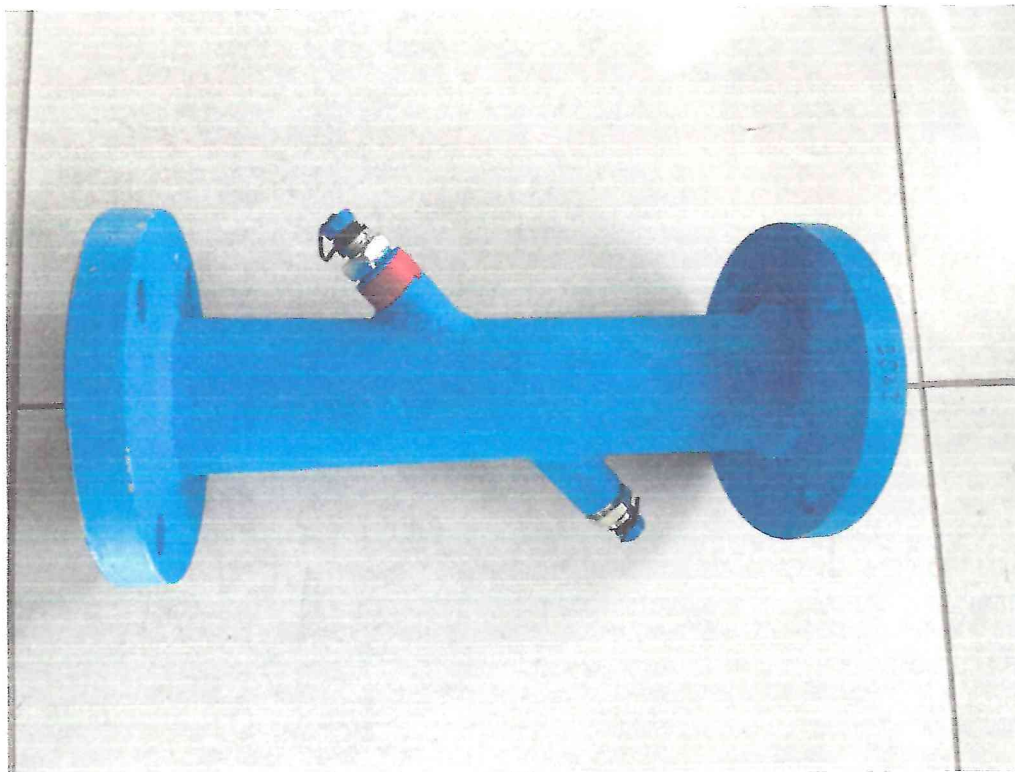
Рисунок 1.2 – Фотография общего вида первичного преобразователя расхода (УПР) расходомера-счетчика ультразвукового РУС-1 № 17285
