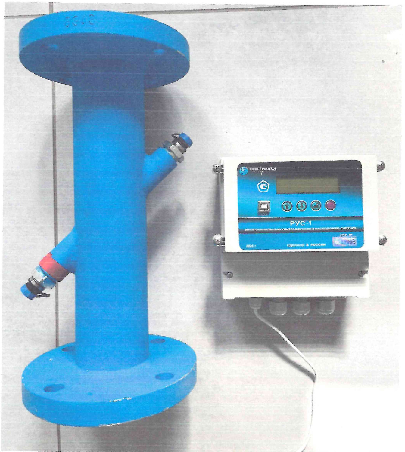
Рисунок 1.1 – Фотография общего вида. Расходомер-счетчик ультразвуковой РУС-1 № 17285
