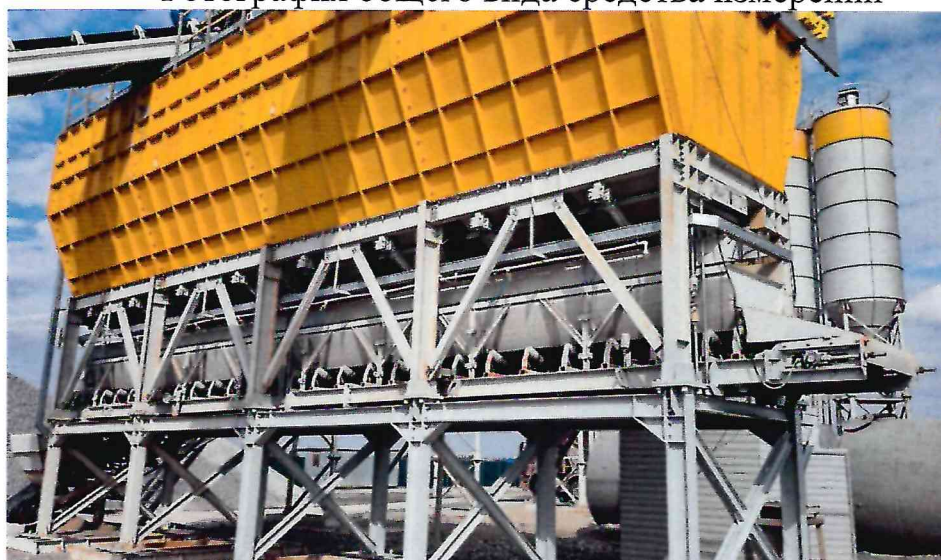
Рисунок 1.1 – Фотография внешнего вида дозатора для инертных материалов ДИ-10000 № ТСУТ-000331 в составе бетонного завода SMARTBETON 135 № 187368
