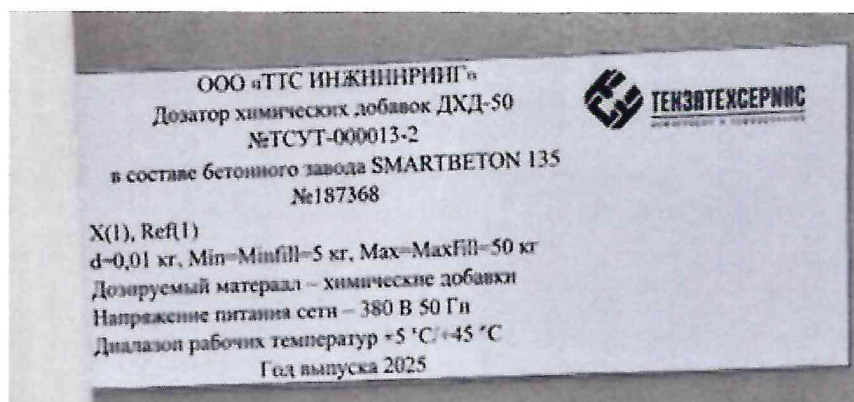
Рисунок 1.2 – Фотография маркировки дозатора химических добавок ДХД-50 № ТСУТ-000013-2 в составе бетонного завода SMARTBETON 135 № 187368
