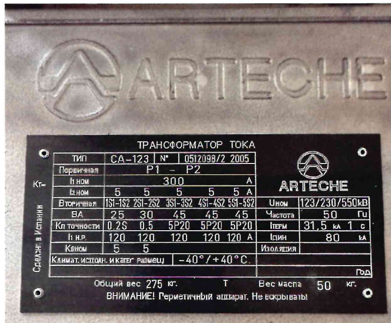
Рисунок 1.2 – Фотография маркировки трансформатора тока СА-123 № 0512098/2
