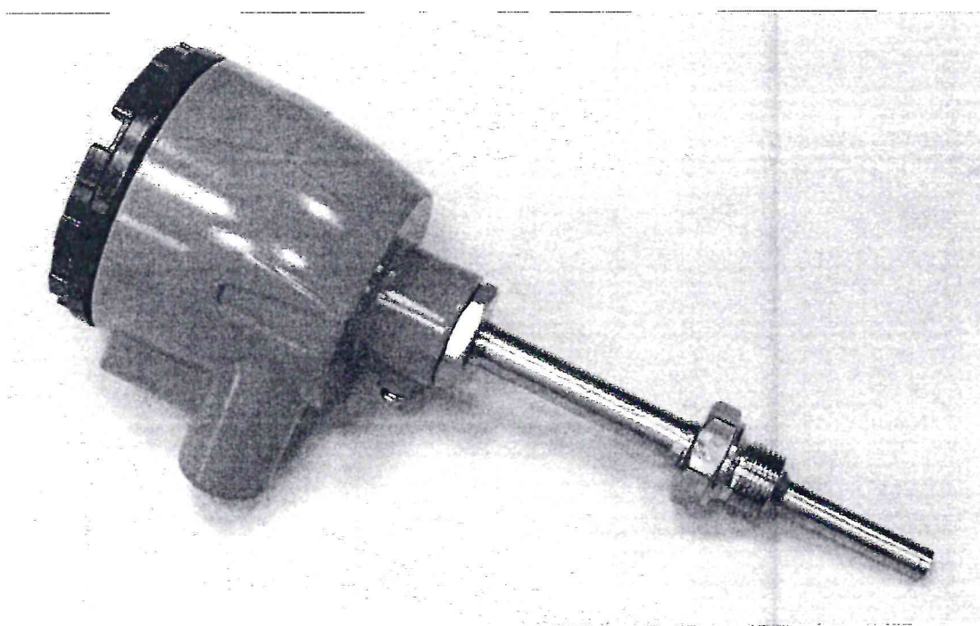
Рисунок 2 – Датчики ТСМУ-Ех(d), ТСПУ-Ех(d), ТХАУ-Ех(d)
