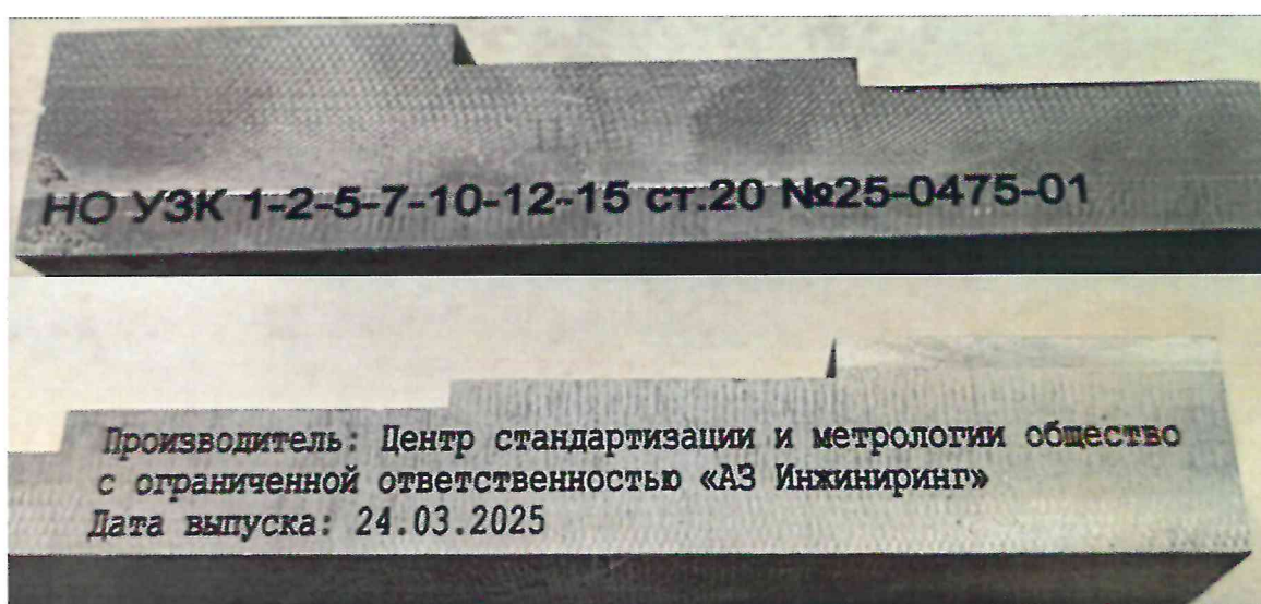
Рисунок 1.2 – Фотография маркировки Настроечного образца НО УЗК – стандартный образец предприятия типа «Ступенька» № 25-0475-01
