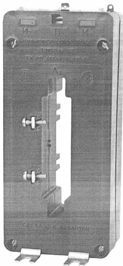
Рисунок 7 – Трансформаторы тока ТШП-0,66У3 на первичные токи 1000, 1500 и 2000 А
