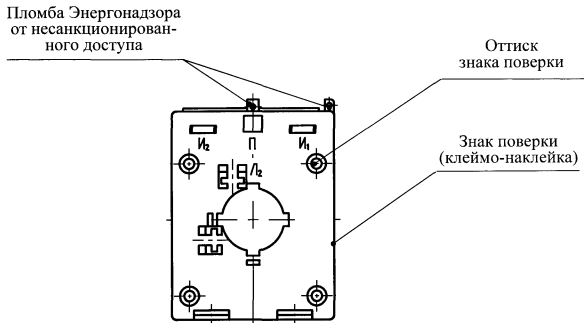
Рисунок А.2 – Трансформаторы тока ТОП-0,66У3 и ТШП-0,66У3
