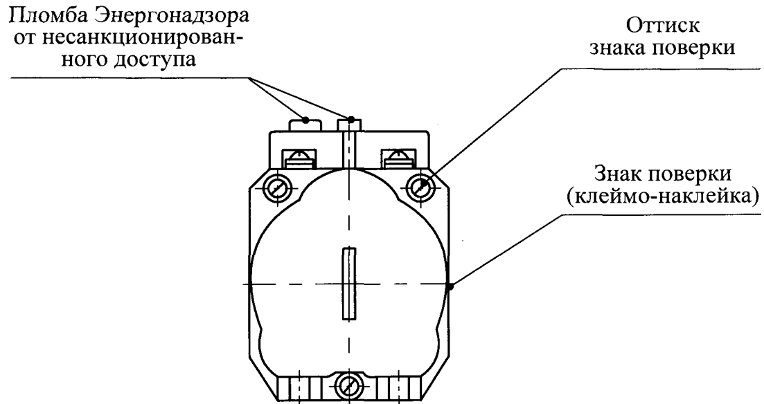
Рисунок А.1 – Трансформаторы тока Т-0,66У3
