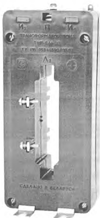
Рисунок 7 – Трансформаторы тока ТИШП-0,66У3 на первичные токи 1000, 1500 и 2000 А
