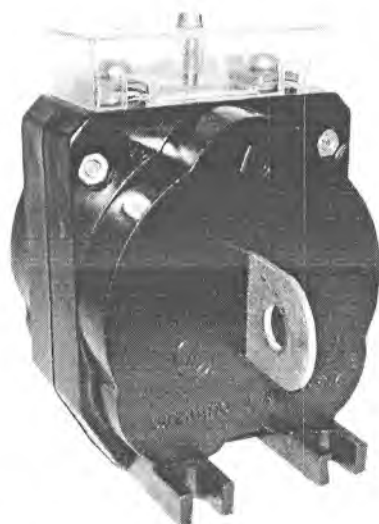
Рисунок 1 – Трансформаторы тока Т-0,66У3 на первичные токи от 10 до 200 А
