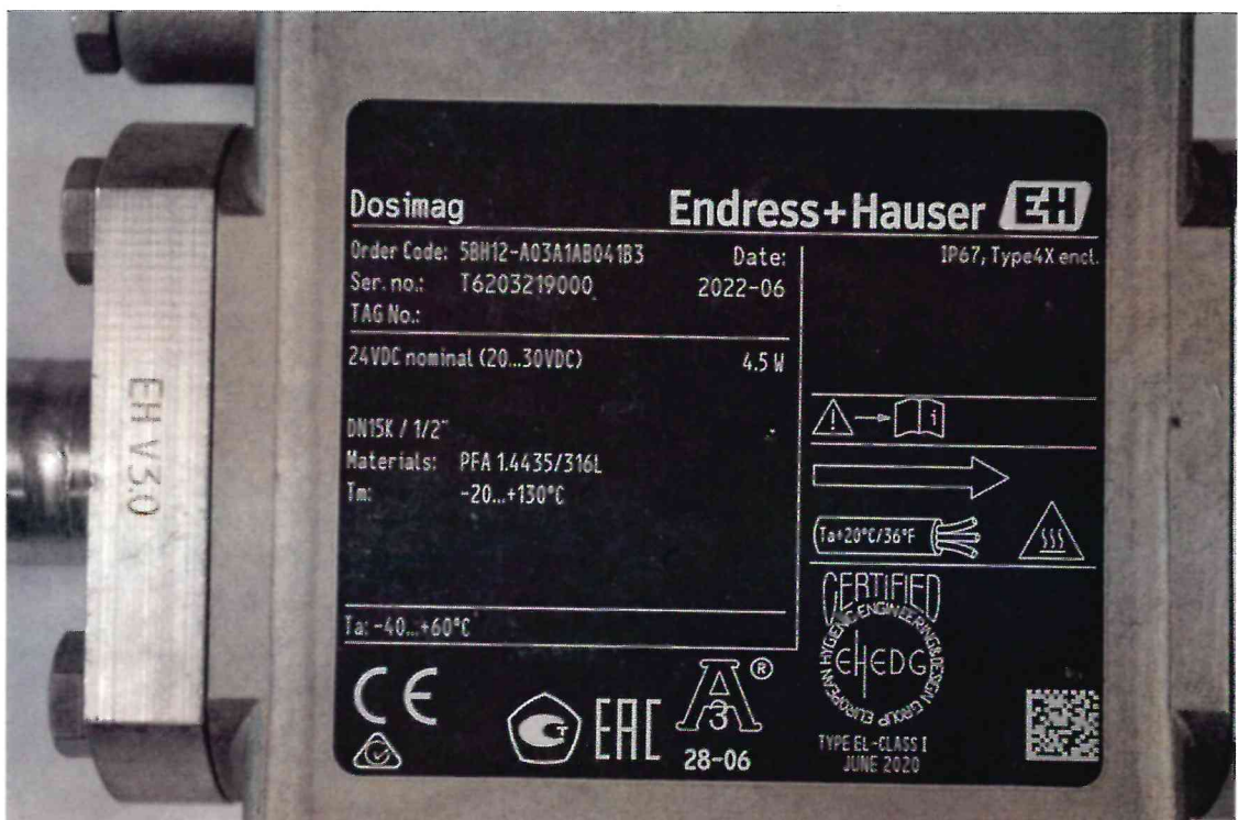
Рисунок 1.2 – Фотография маркировки расходомера электромагнитного Dosimag № T6203219000
