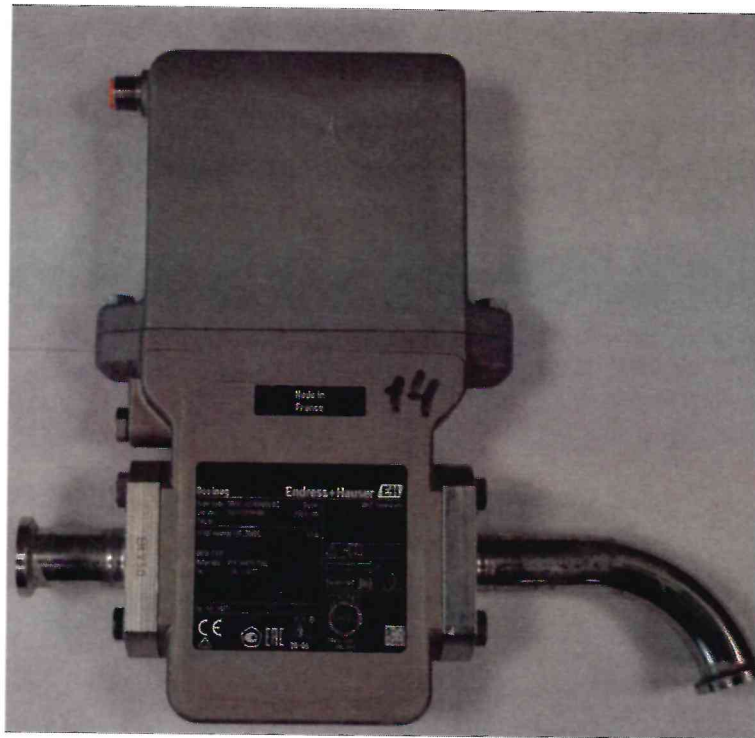
Рисунок 1.1 – Фотография общего вида расходомера электромагнитного Dosimag № T6203519000
