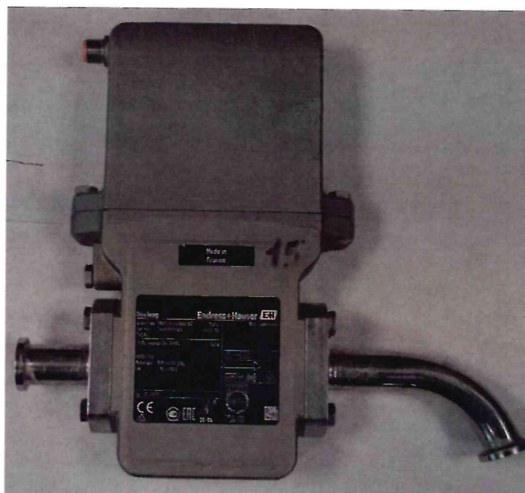
Рисунок 1.1 – Фотография общего вида расходомера электромагнитного Dosimag № T6203119000
