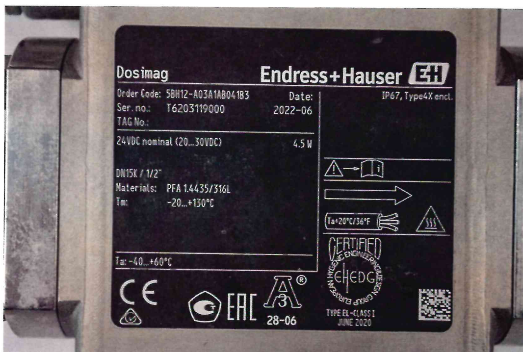
Рисунок 1.2 – Фотография маркировки расходомера электромагнитного Dosimag № T6203119000
