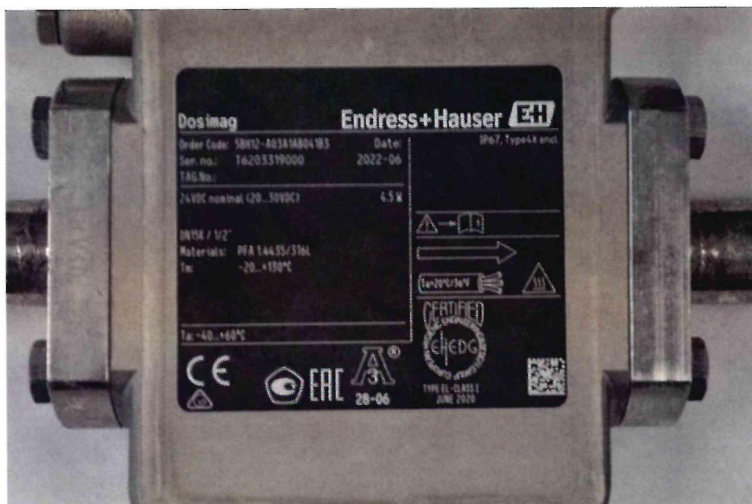
Рисунок 1.2 – Фотография маркировки расходомера электромагнитного Dosimag № T6203319000
