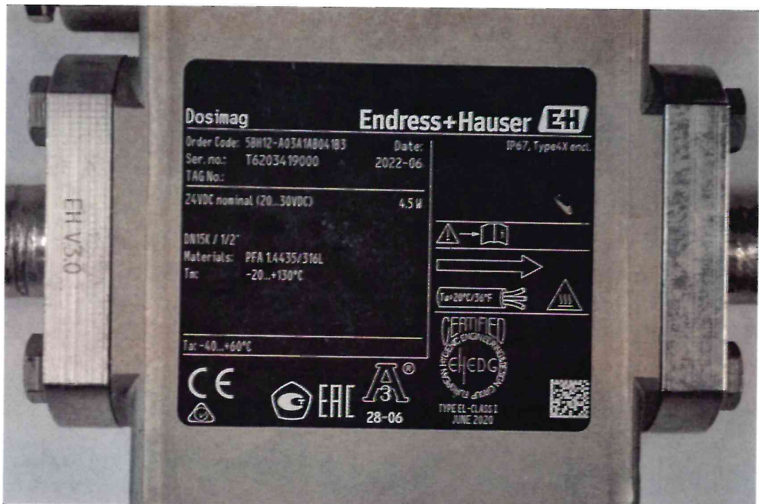
Рисунок 1.2 – Фотография маркировки расходомера электромагнитного Dosimag № T6203419000
