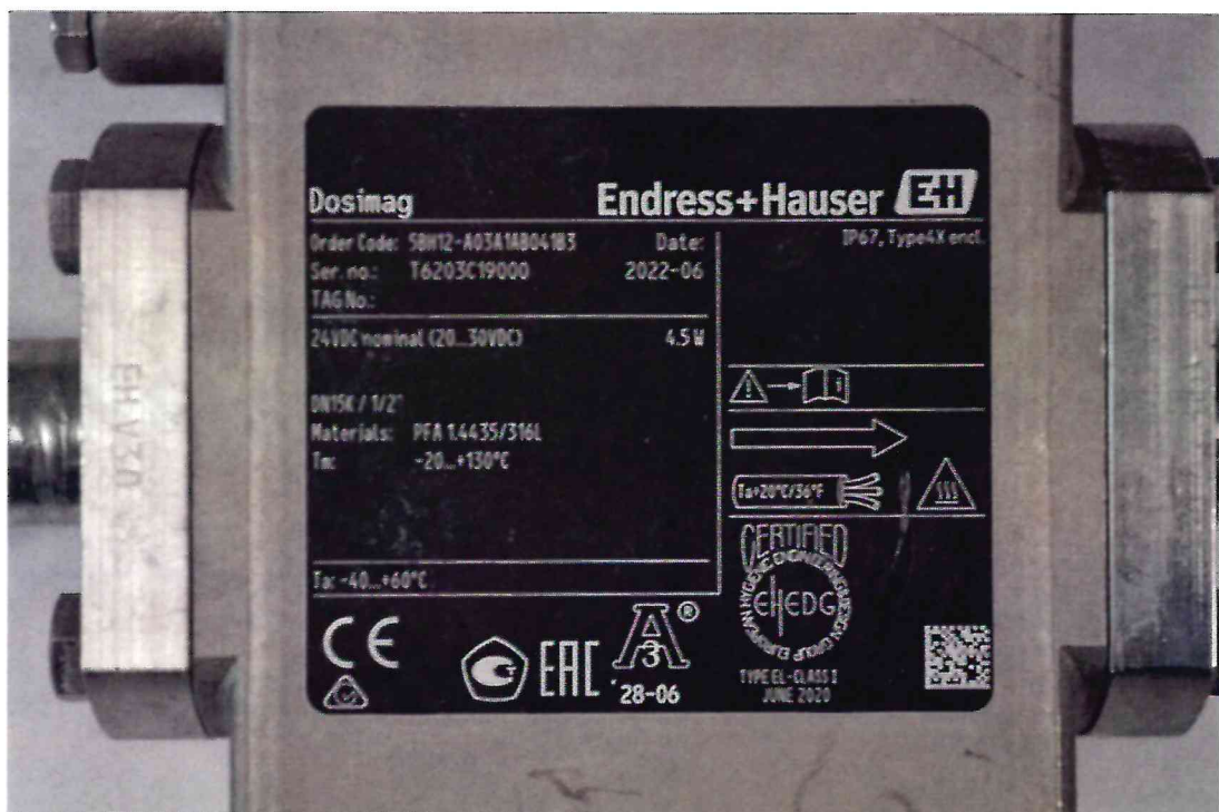
Рисунок 1.2 – Фотография маркировки расходомера электромагнитного Dosimag № T6203C19000
