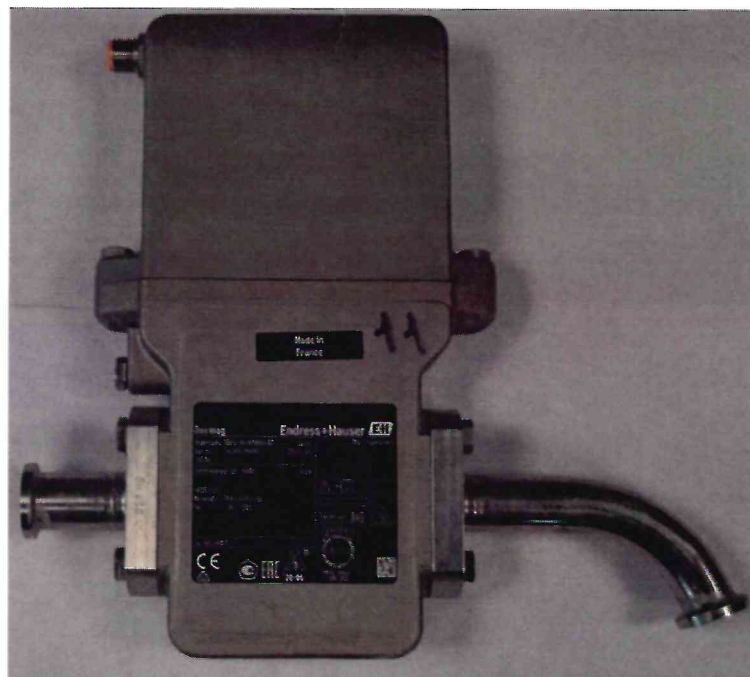
Рисунок 1.1 – Фотография общего вида расходомера электромагнитного Dosimag № T6203C19000
