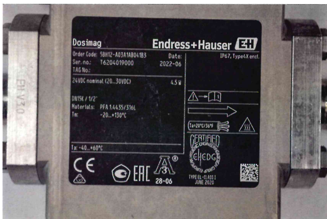
Рисунок 1.2 – Фотография маркировки расходомера электромагнитного Dosimag № T6204019000
