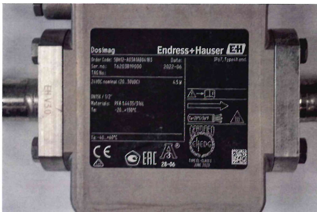
Рисунок 1.2 – Фотография маркировки расходомера электромагнитного Dosimag № T6203B19000
