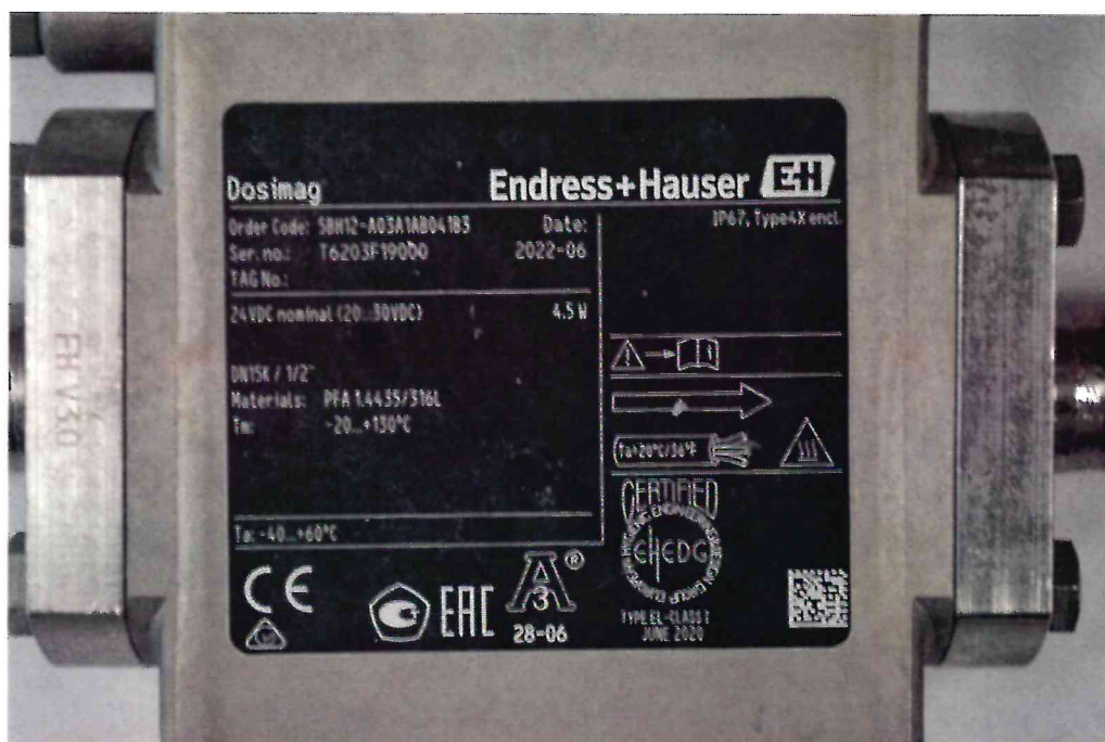
Рисунок 1.2 – Фотография маркировки расходомера электромагнитного Dosimag № T6203F19000
