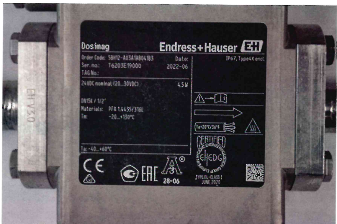
Рисунок 1.2 – Фотография маркировки расходомера электромагнитного Dosimag № T6203E19000
