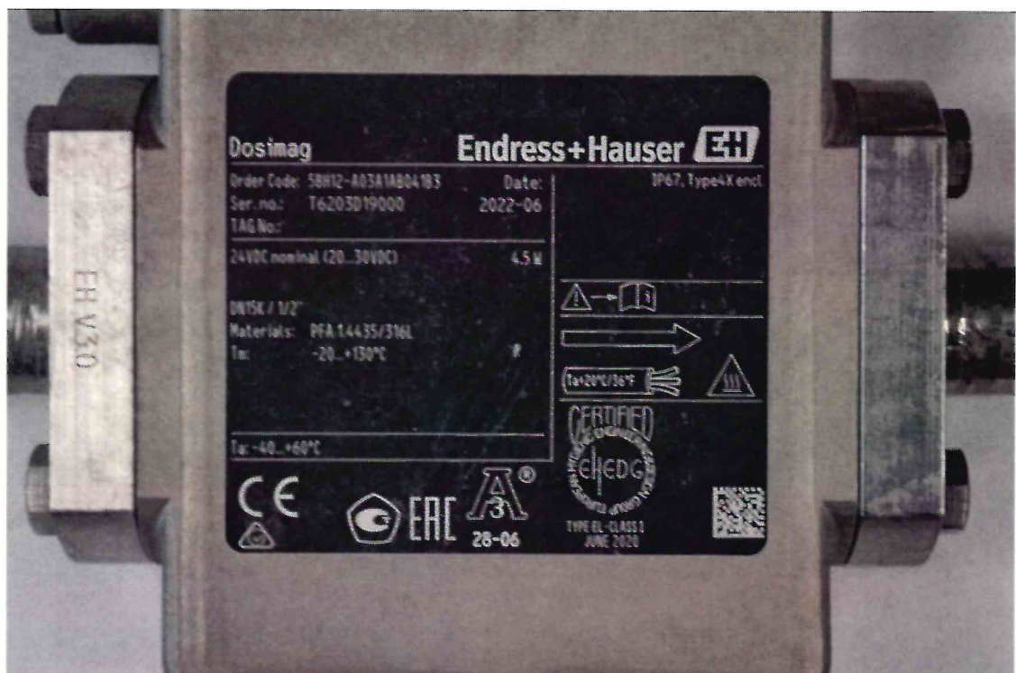
Рисунок 1.2 – Фотография маркировки расходомера электромагнитного Dosimag № T6203D19000
