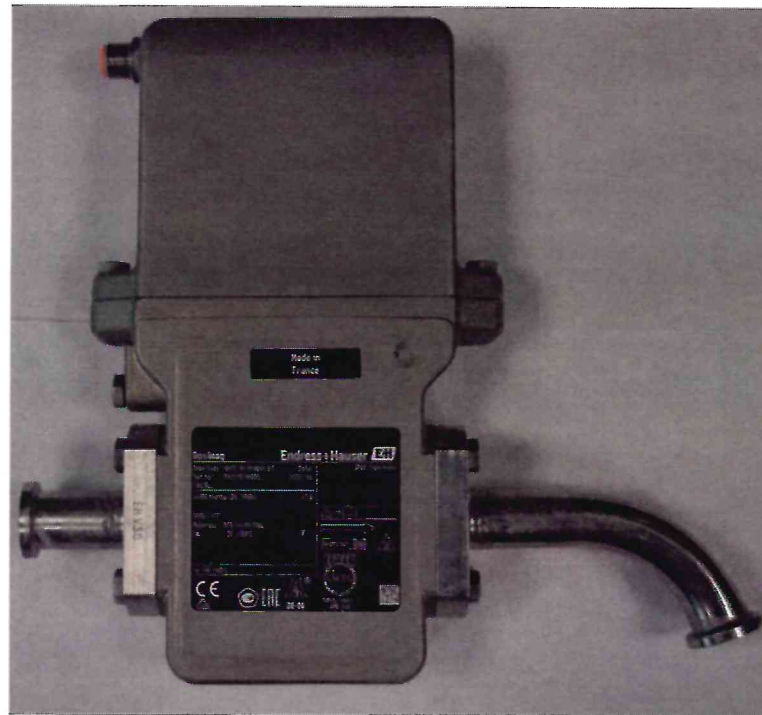
Рисунок 1.1 – Фотография общего вида расходомера электромагнитного Dosimag № T6203D19000
