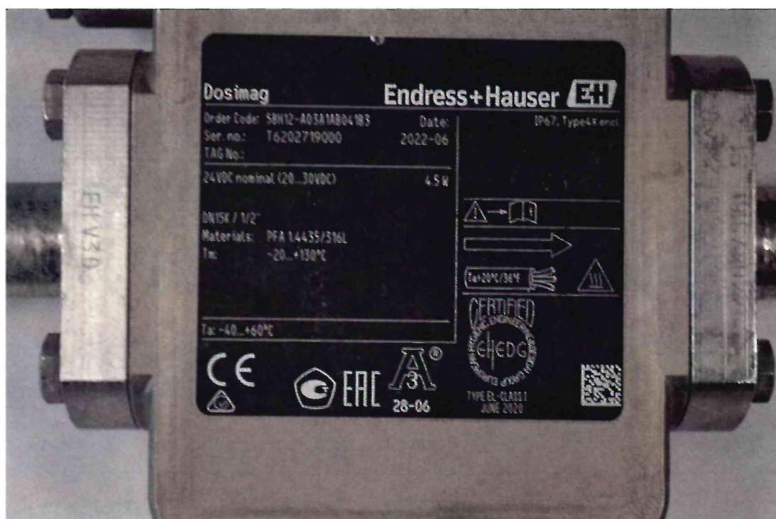
Рисунок 1.2 – Фотография маркировки расходомера электромагнитного Dosimag № T6202719000
