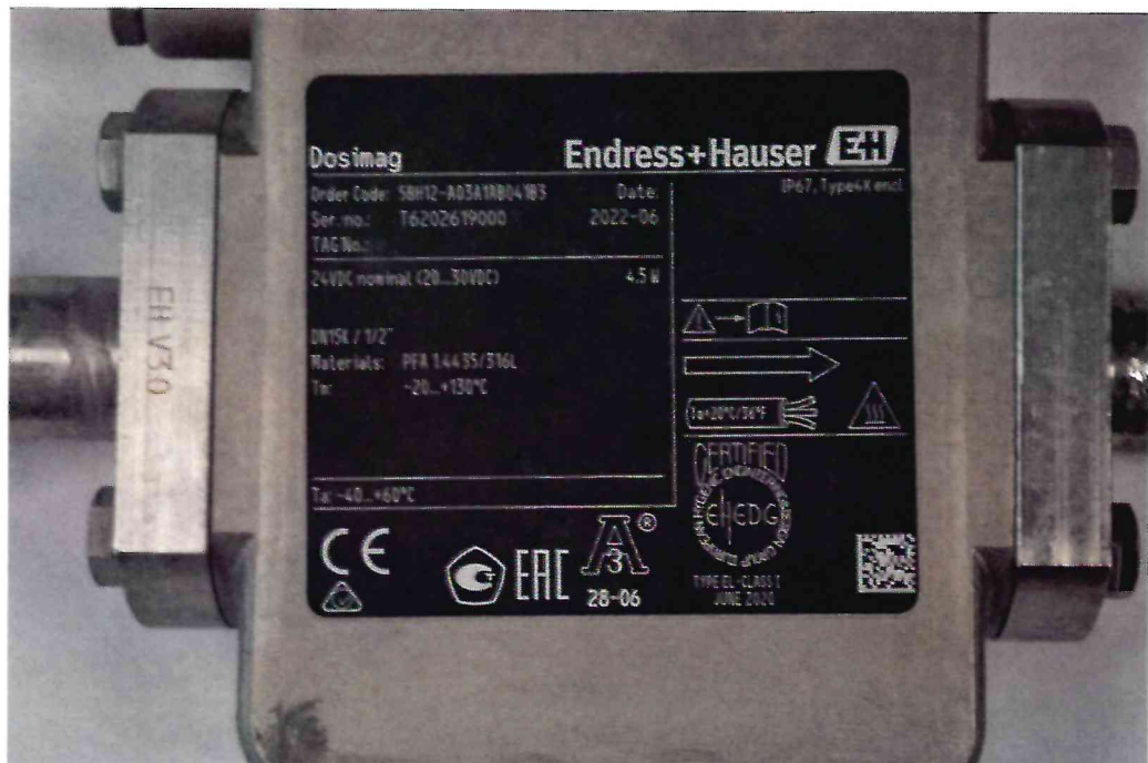
Рисунок 1.2 – Фотография маркировки расходомера электромагнитного Dosimag № T6202619000
