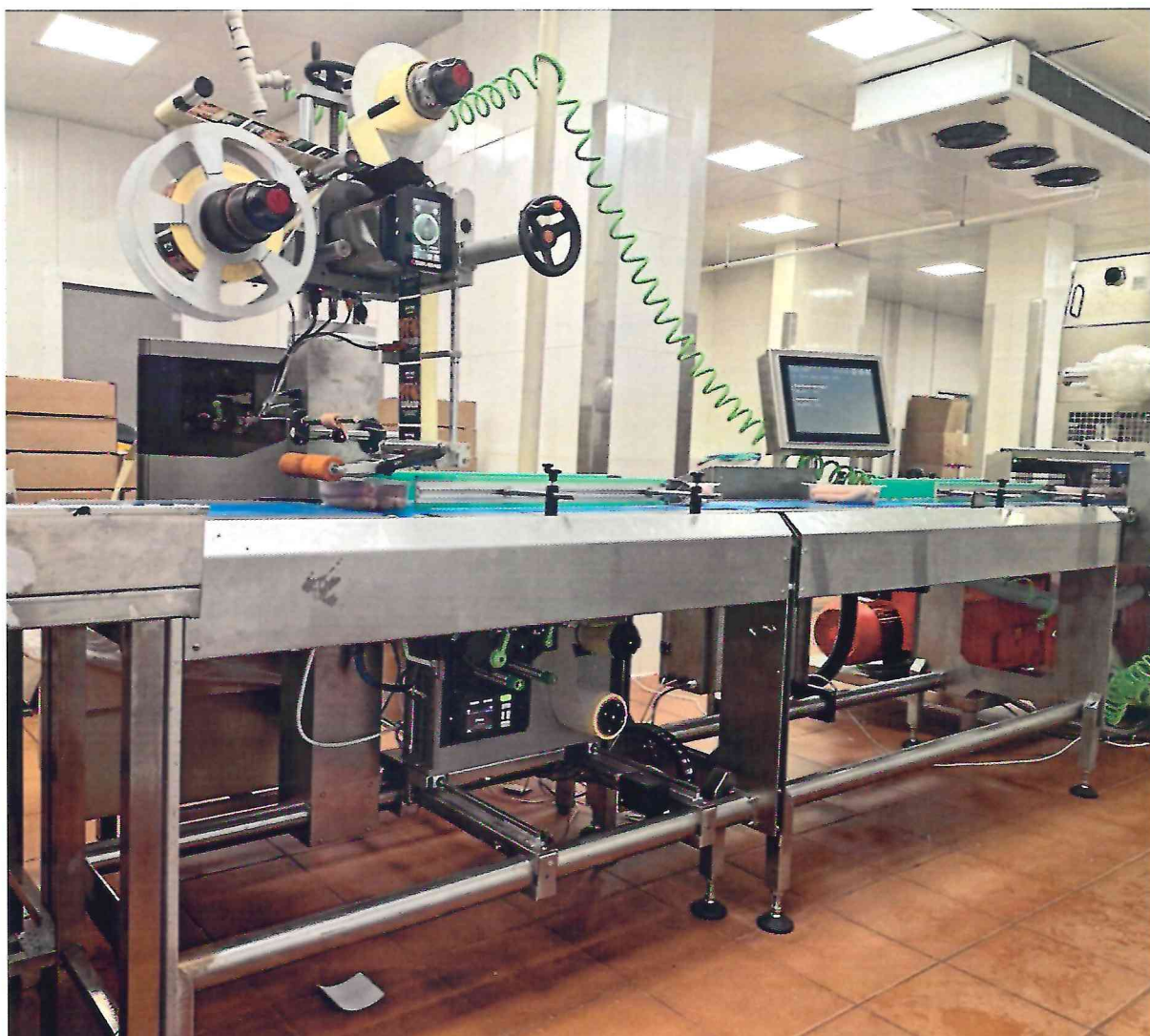
Рисунок 1.1 – Фотографии общего вида автоматического весового этикетировочного комплекса WS-6 № 1232522
