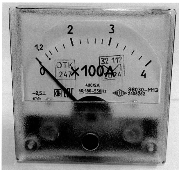
Рисунок 3 - Общий вид амперметров Э8030-М1Э экспортное исполнение
