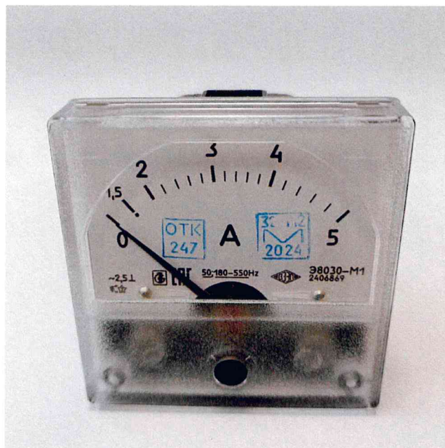
Рисунок 1 - Общий вид амперметров Э8030-М1 обычного исполнения
