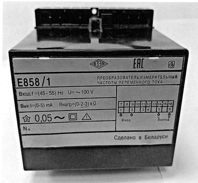
Рисунок 1 – Общий вид и маркировка ИП E858/1 для нужд народного хозяйства
