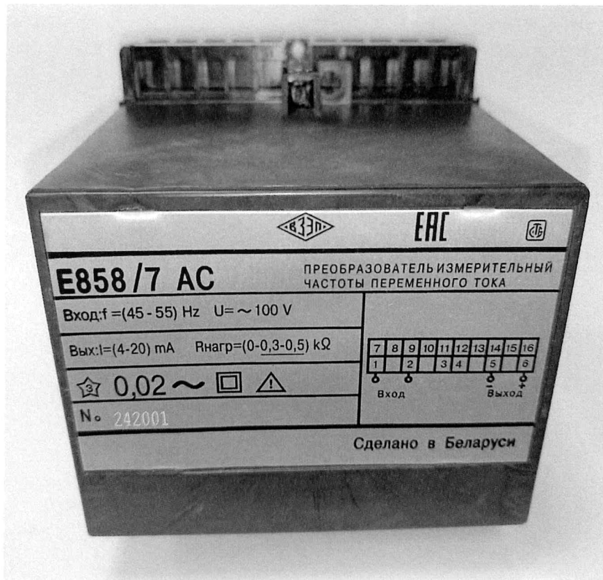
Рисунок 7 – Общий вид и маркировка ИП E858/7 AC для поставки на атомные станции
