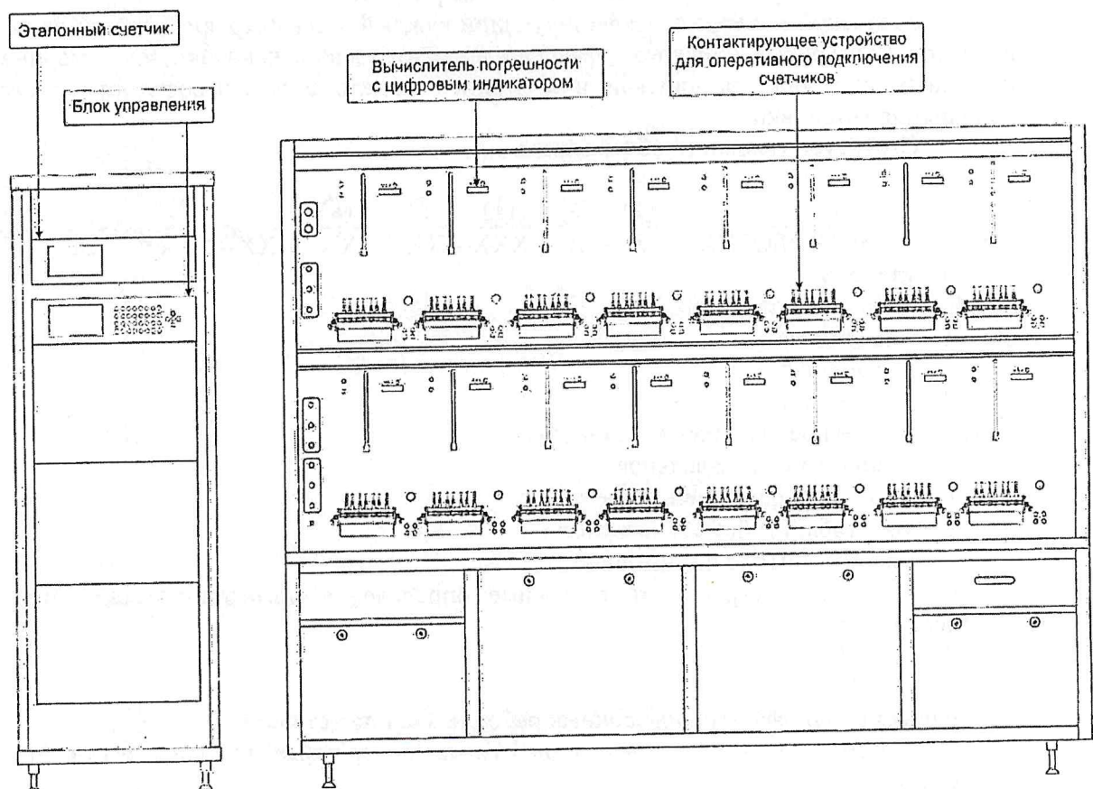
Рисунок 1 – Общий вид установки стационарного раздельного конструктивного исполнения (трехфазной модификации на 16 рабочих мест)
