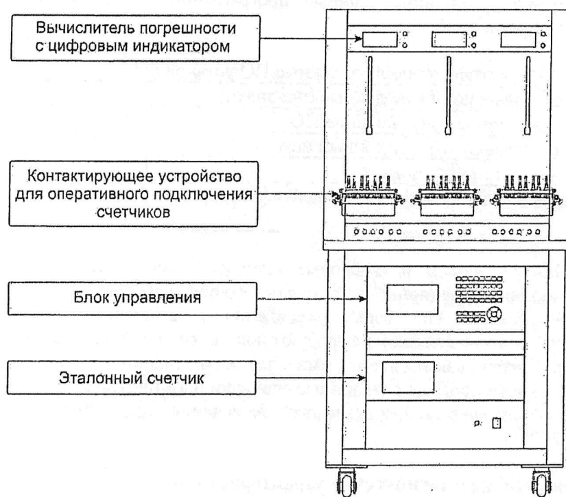
Рисунок 3 – Общий вид установки малогабаритного лабораторного конструктивного исполнения (трехфазной модификации на 3 рабочих места)
