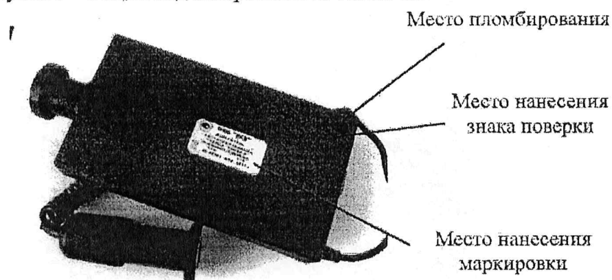
Рисунок 1 – Общий вид измерителей «ТОНИК-Н»
