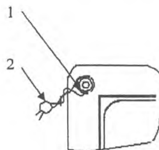
Рисунок. 2 - Схема пломбировки расходомеров-счетчиков ультразвуковых «ВЗЛЕТ РСЛ»
