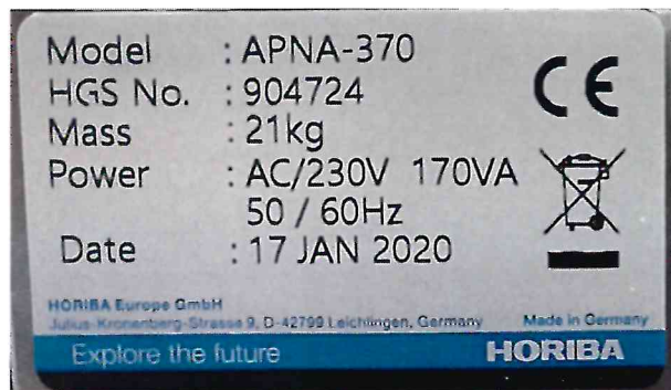
Рисунок 1.2 – Фотография маркировки анализатора окислов азота APNA-370 № 904724
