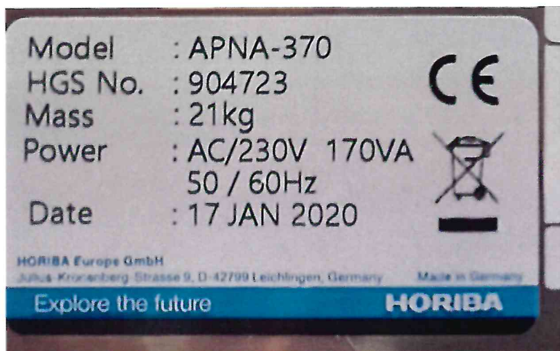
Рисунок 1.2 – Фотография маркировки анализатора окислов азота APNA-370 № 904723
