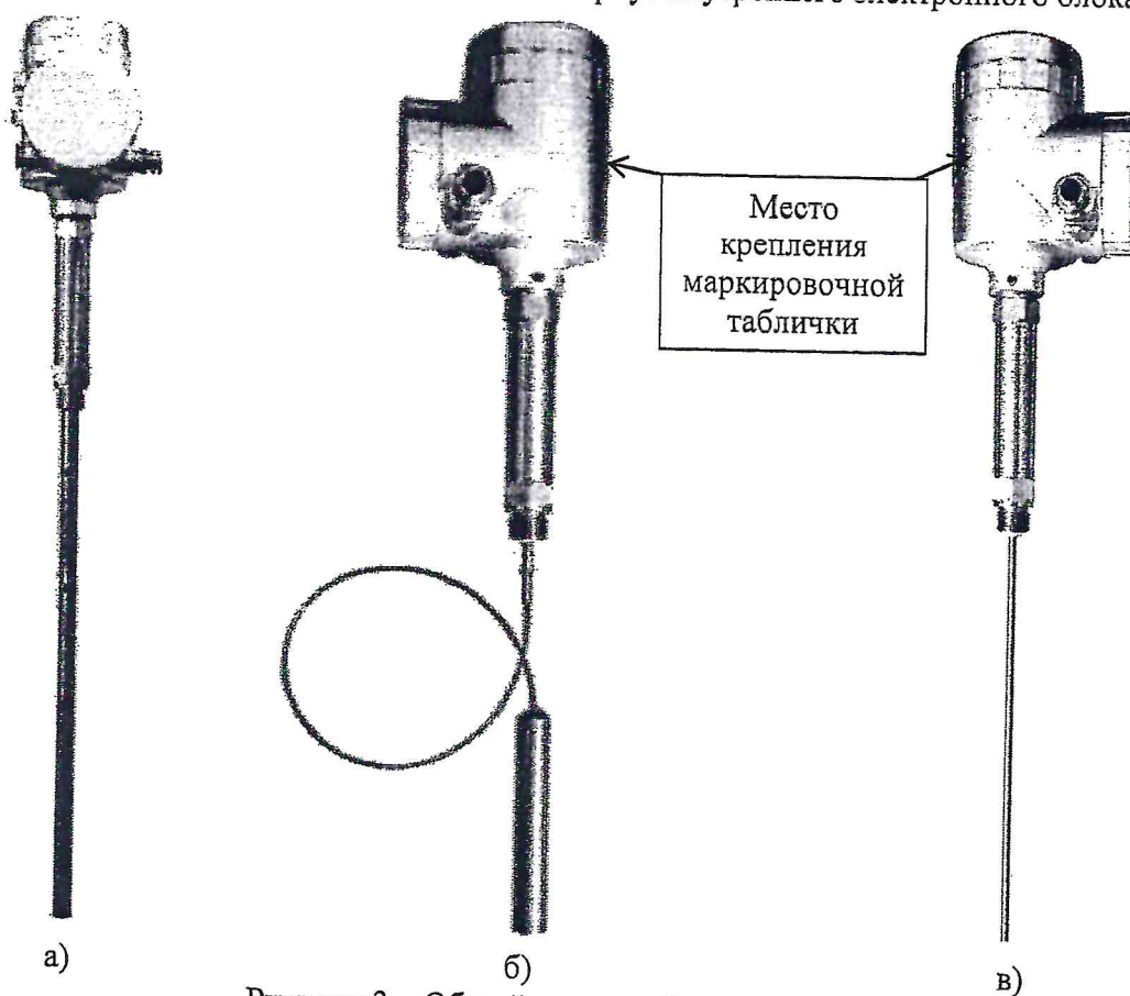
Рисунок 3 – Общий вид преобразователей
