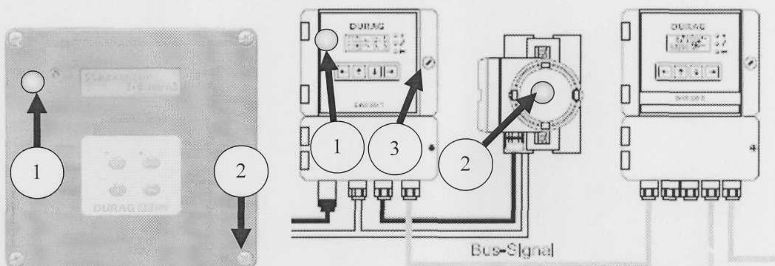
Схема 4 Расположение клейма-наклейки (1) на электронном блоке BR800PR00, BR800PR10 установки D-R 800 и место пломбировки прибора (2)
