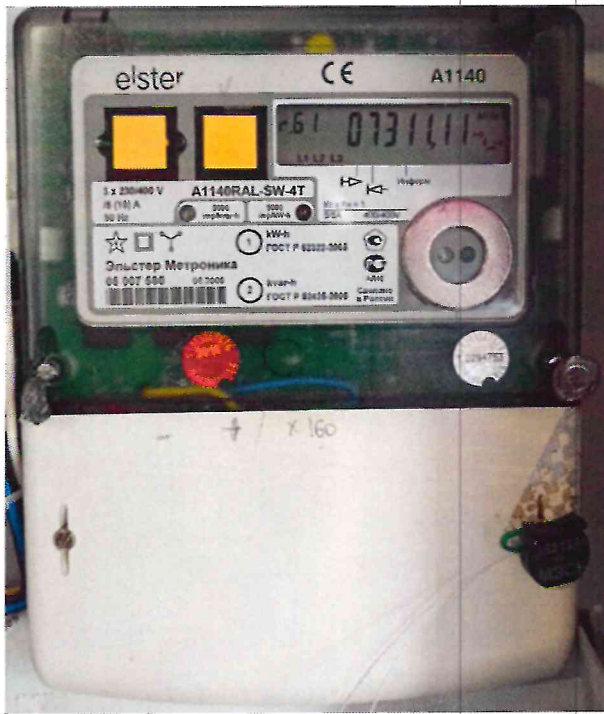
Рисунок 1.2 – Фотографии счётчиков, входящих в состав измерительных каналов АСКУЭ (изображения носят иллюстративный характер)
