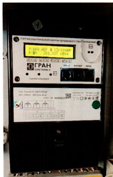
Измерительный канал № 2
