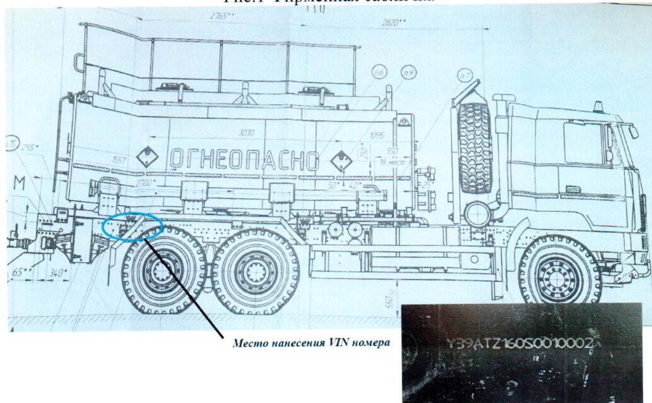
Рис.2 Маркировка идентификационного номера, расположенного на правом лонжероне шасси
