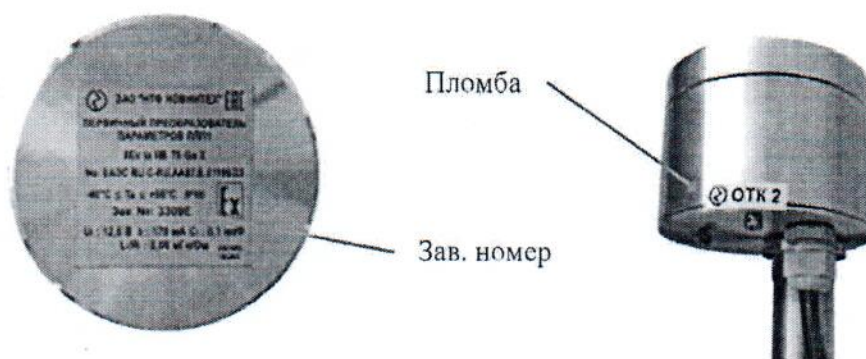
Рисунок 16 – Внешний вид ППП(контроллер)
