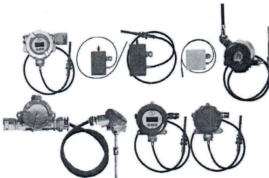
Рисунок 3 – Общий вид погружаемых кабельных общепромышленных ППТСК/Оп, ППТСК/Оп/ИНД и взрывозащищенных ППТСК/Exi, ППТСК/Exi/ИНД
