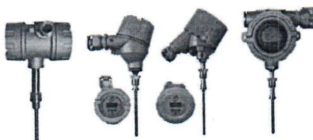
Рисунок 2 – Общий вид погружаемых общепромышленных ППТС/Оп/ИНД и взрывозащищенных ППТС/Exd/ИНД, ППТС/Exi/ИНД, ППТС/Exdi/ИНД
