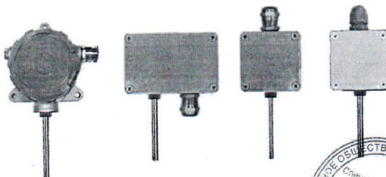
Рисунок 4 – Общепромышленные ТСп-Оп и взрывозащищенные ТСп-Ехi для измерений температуры окружающей среды (воздуха)
