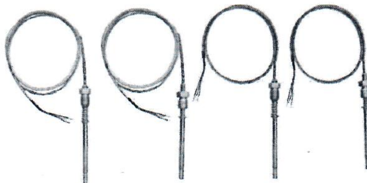
Рисунок 3 – Общепромышленные TCM 321M-Op, TСП 321M-Op и взрывозащищенные TCM 321M-Exi, TСП 321M-Exi
