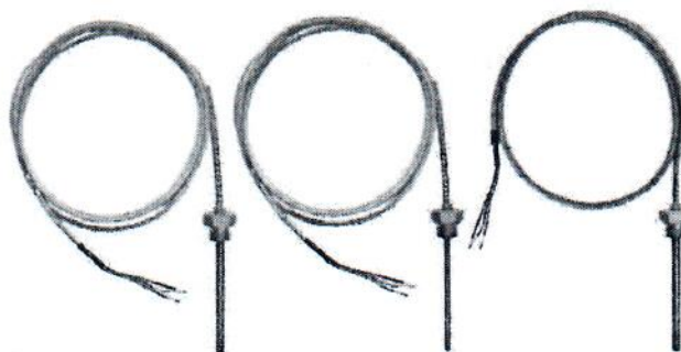
Рисунок 4 – Общепромышленные TCM 322M-Op, TСП 322M-Op и взрывозащищенные TCM 322M-Exi, TСП 322M-Exi
