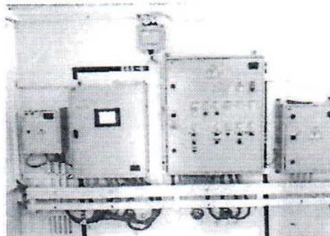
Рисунок 5 – Внешний вид оборудования БА общепромышленного исполнения
