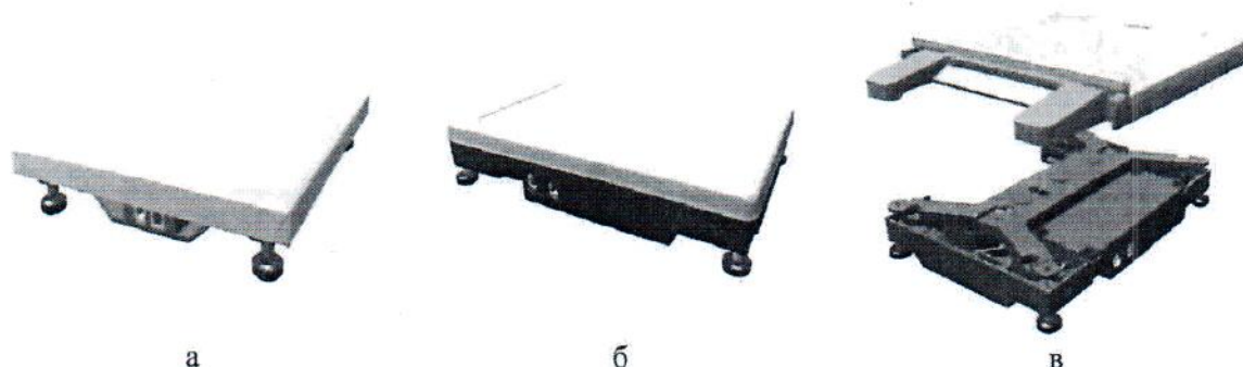
Рисунок 2 – Общий вид модуля:
