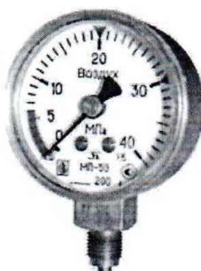
Манометры показывающие МП для дыхательных аппаратов
