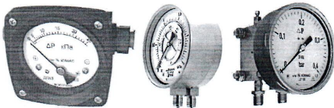
Дифманометры показывающие ДП, в т. ч. взрывозащищенные
